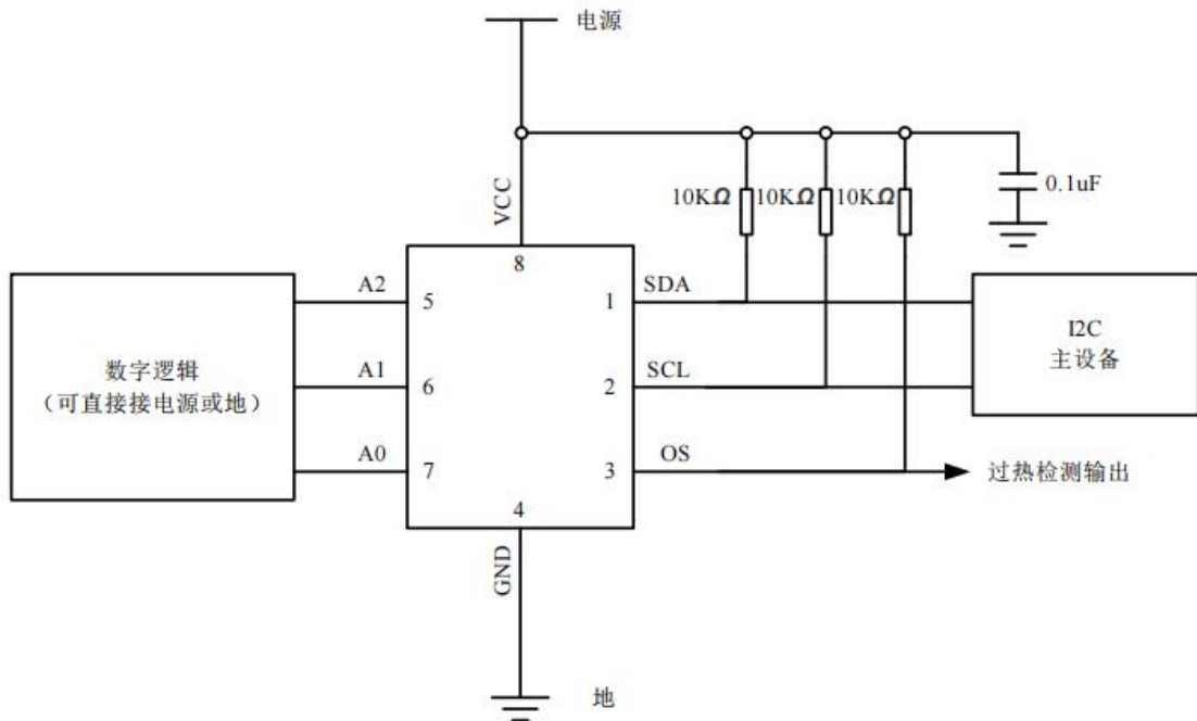
图 3-1 典型应用图
