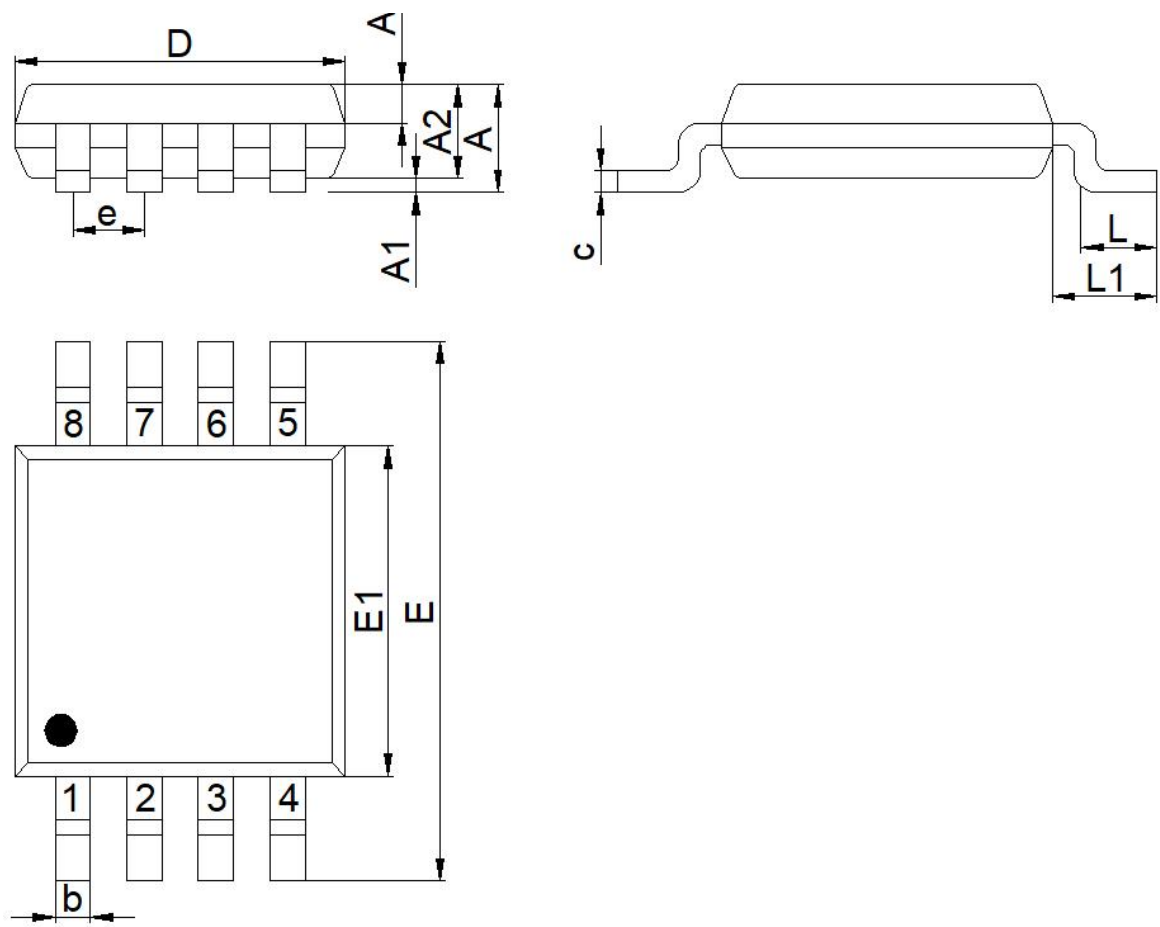
VSS0P8 封装外形尺寸
