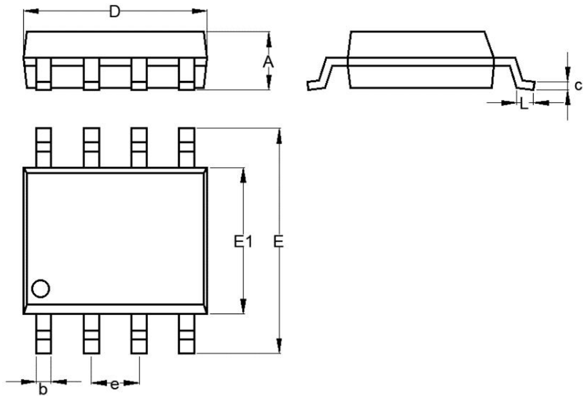
SOP-8 外形图
