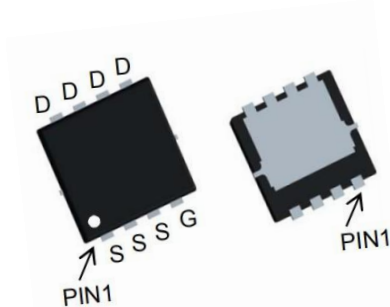
PDFN3X3
