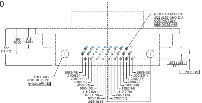
2H26 26 #22
