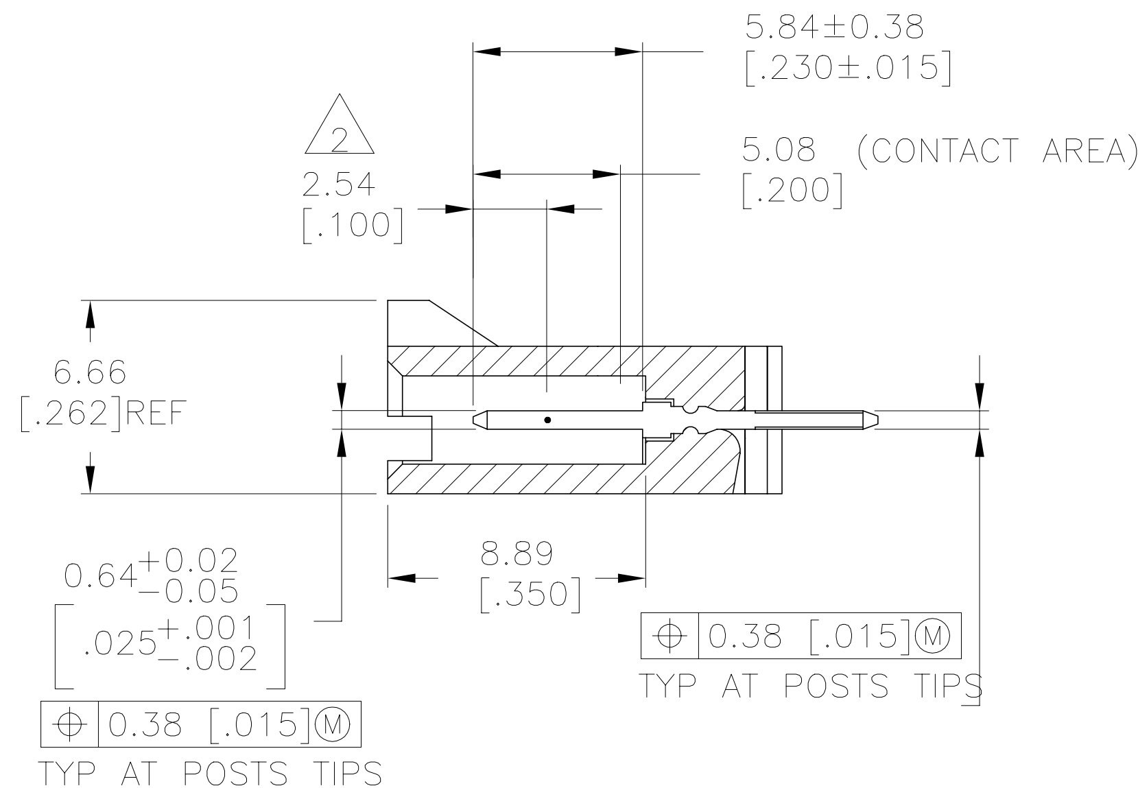
SECTION A-A
