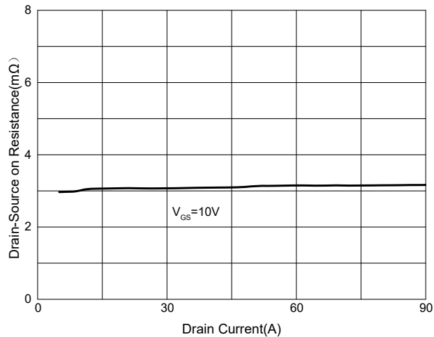
Fig. 4 - R_{DS(ON)} - I_D
