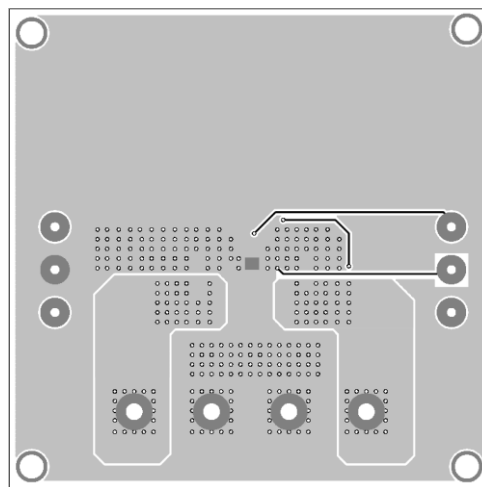
Figure 2—Bottom Layer
