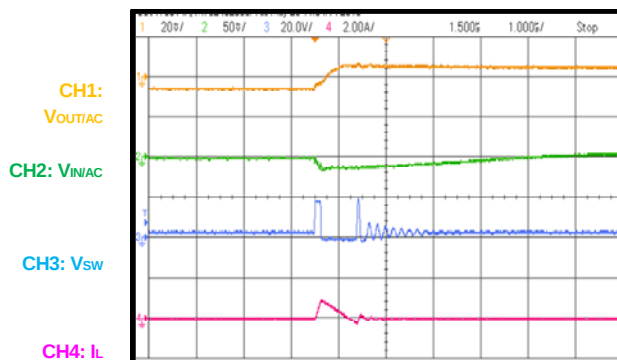
Input/Output Ripple I_{OUT} = 0A , USM
