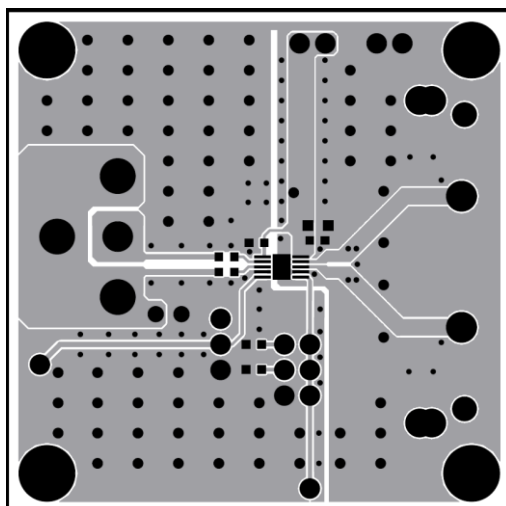
Figure 1—Top Layer
