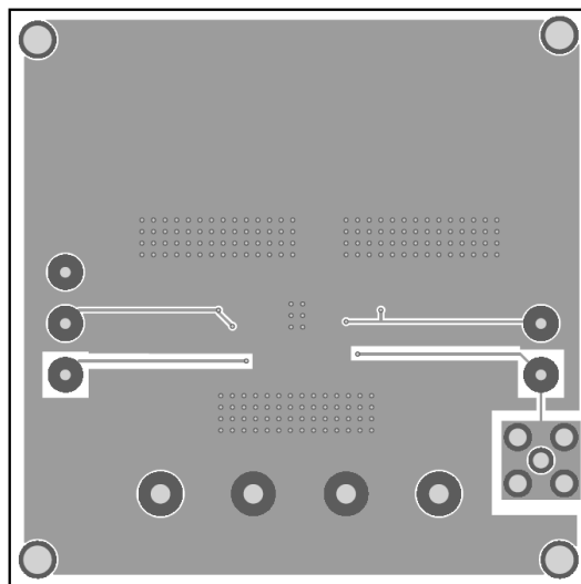
Figure 2—Bottom Layer
