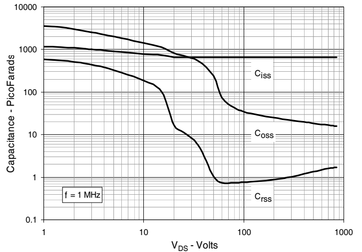
Fig. 12. Capacitance
