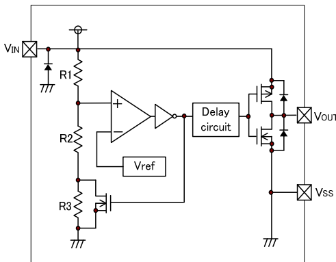
(1) CMOS output
