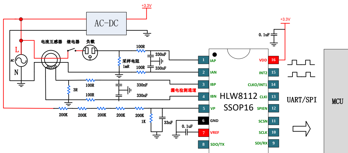
图 5 HLW8112 典型应用图
