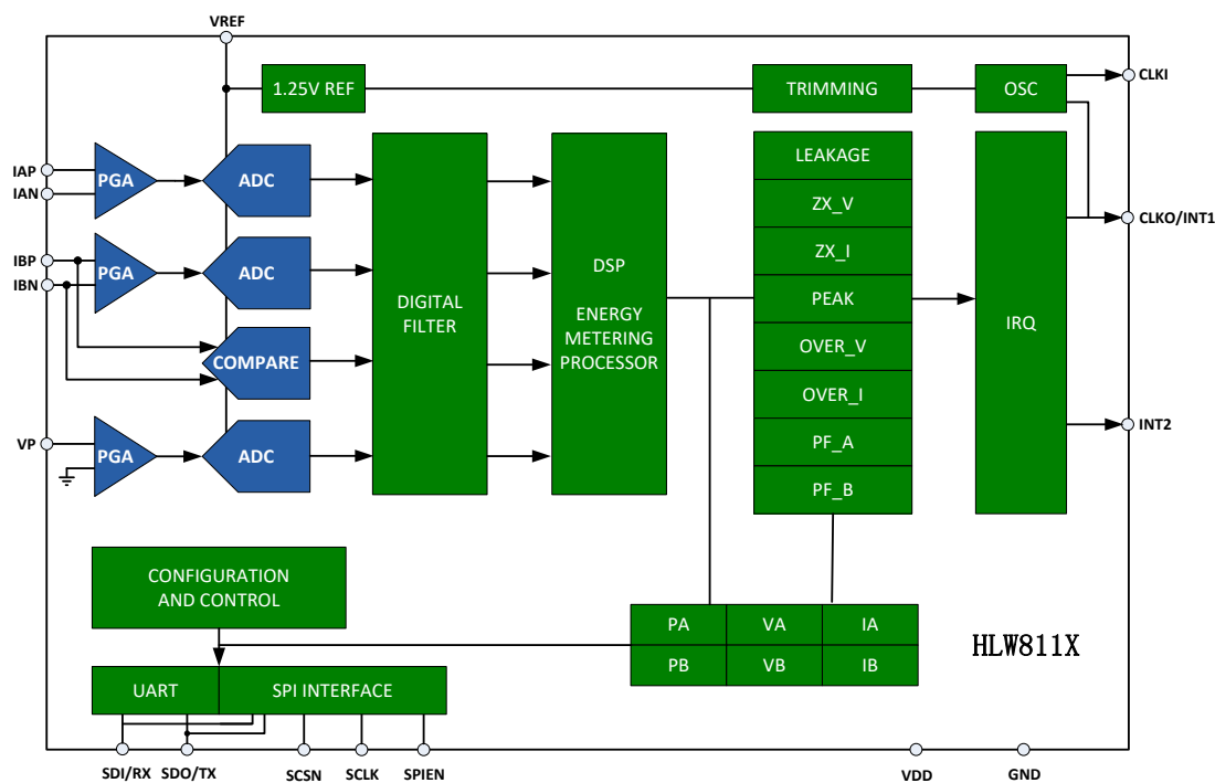
图 1 功能框图
