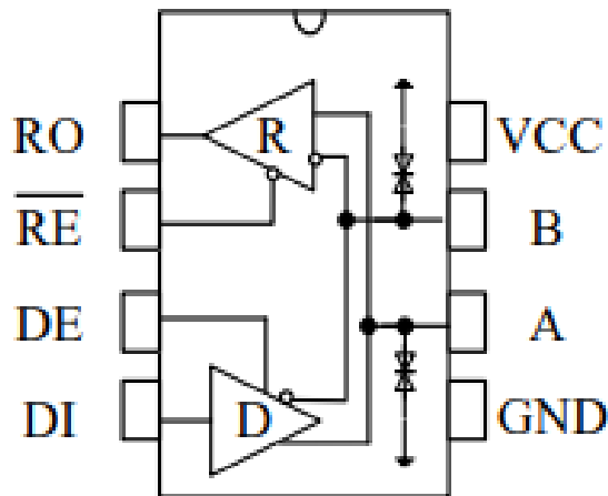
图 1 ES8485E-SR 引脚分布图
