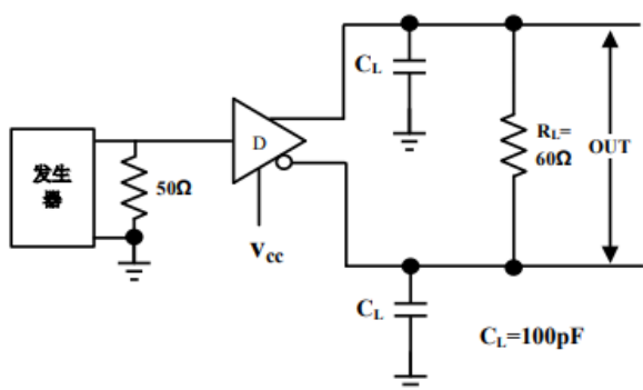
图 2 驱动器直流测试负载
