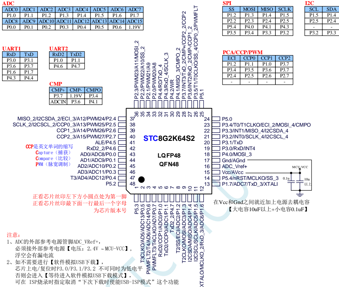
STC8G2K64S2-36I-LQFP48/QFN48 最小系统 示意图
