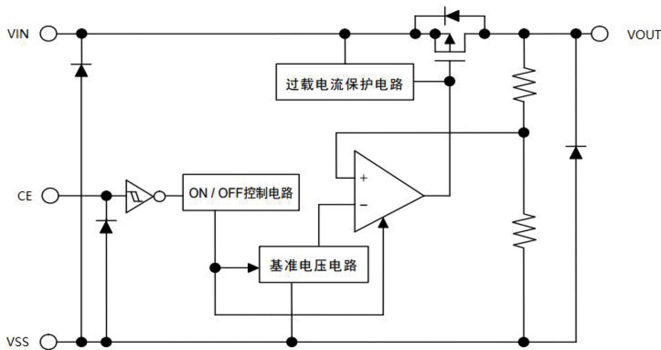
电路方框图
