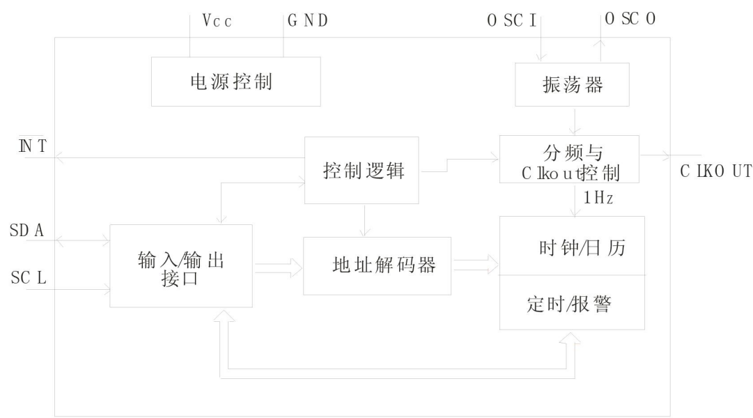
图 2. 方框图
