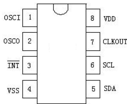
图 3. 引脚图
