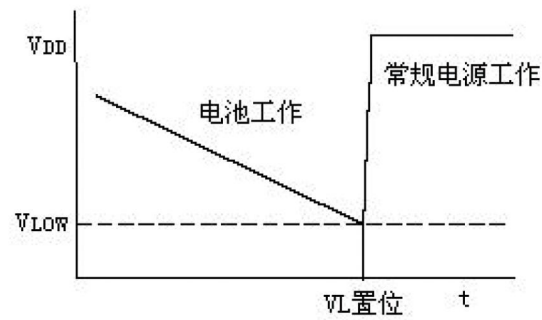
图8. 掉电检测
