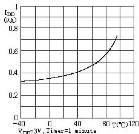
CLKOUT=32.768kHz, I_{DD} 与 T_A 关系图
