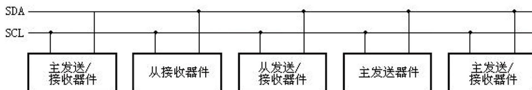
图10. I2C总线系统配置图
