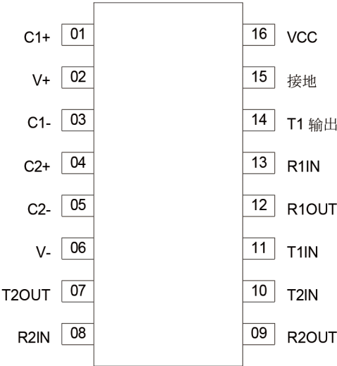
SOP -16 PKG
