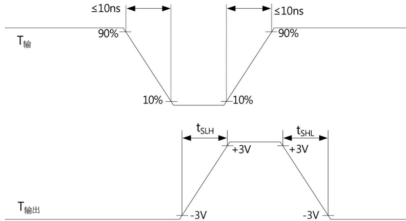
图 3. t_{SLH} 和 t_{SHL} 发射机波形
