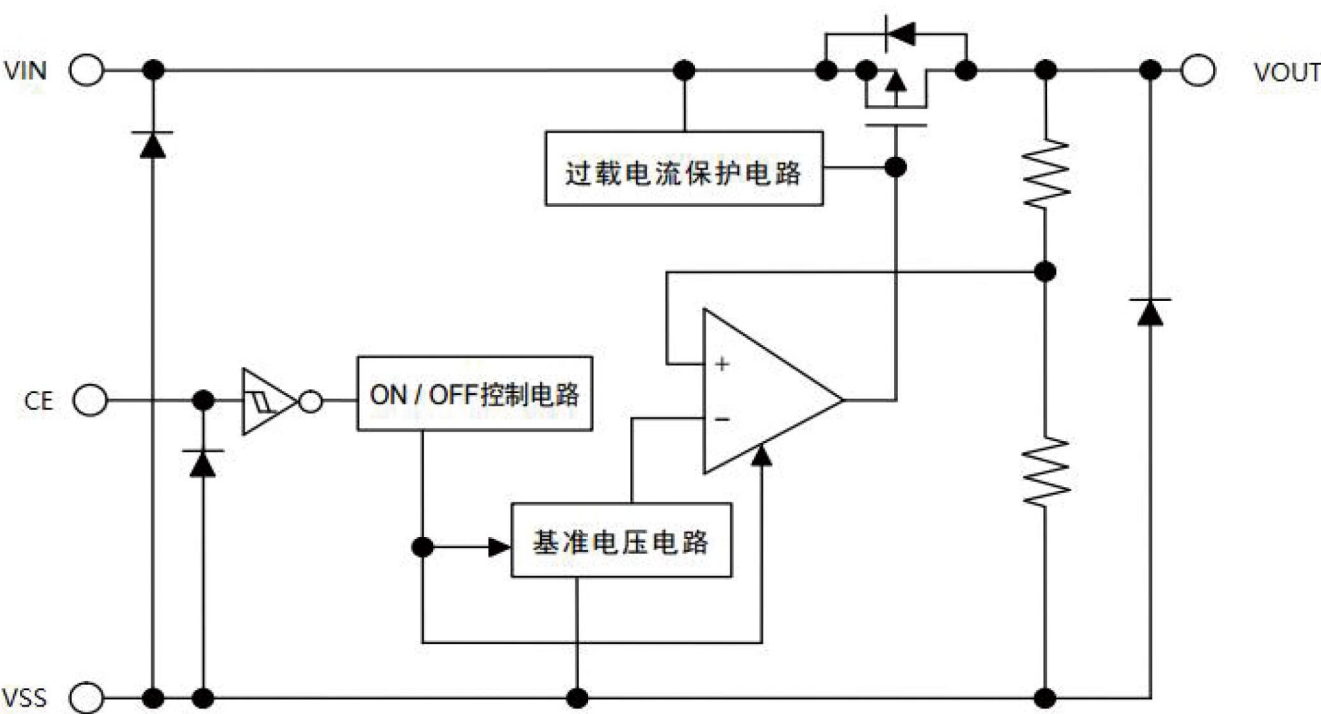
电路方框图
