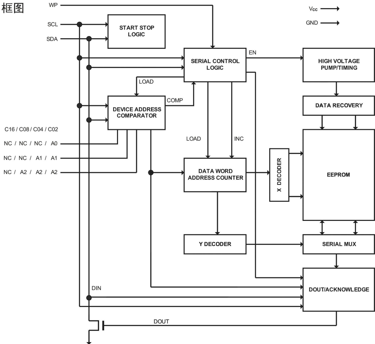
图1 框图
