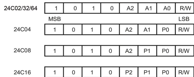
图8 器件地址
