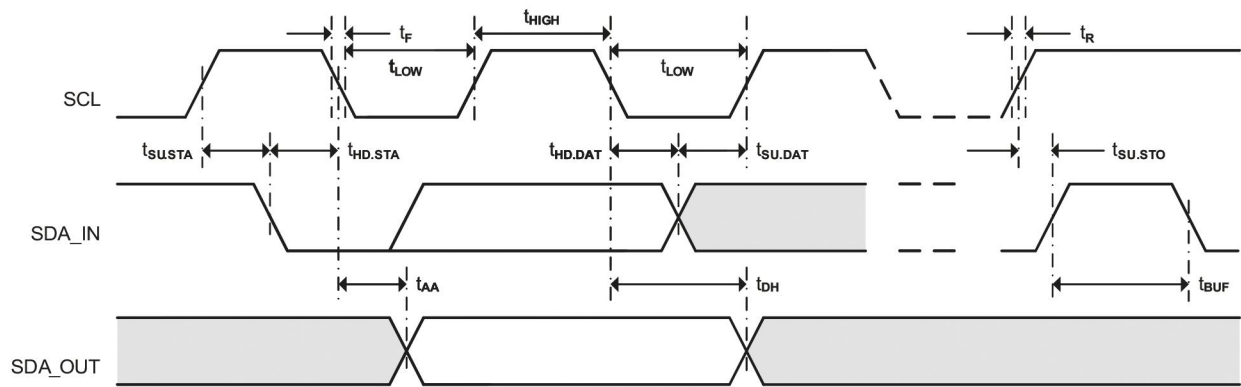
图2 总线时序
