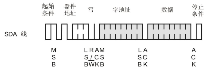
图9 字节写
