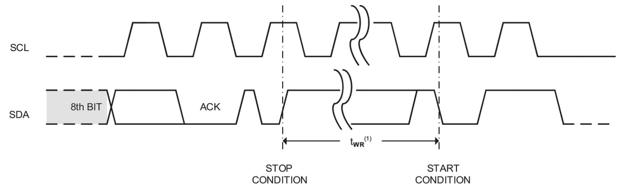
图2 总线时序
