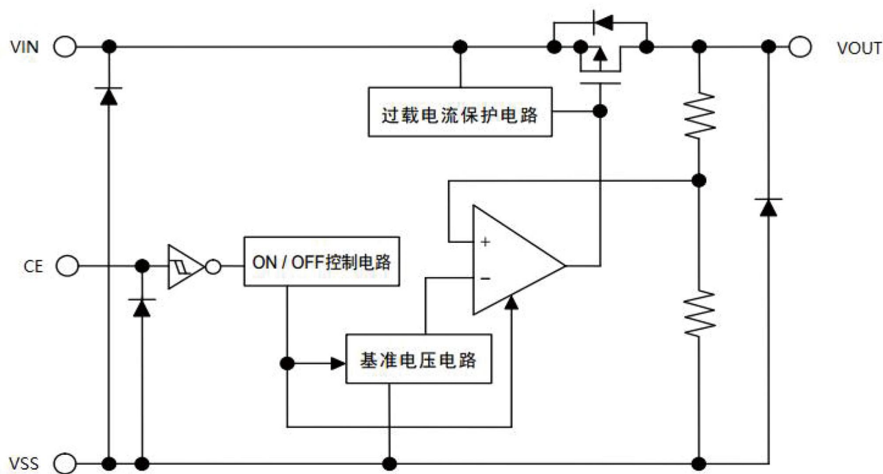
电路方框图
