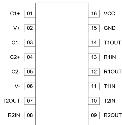
SOP -16 PKG
