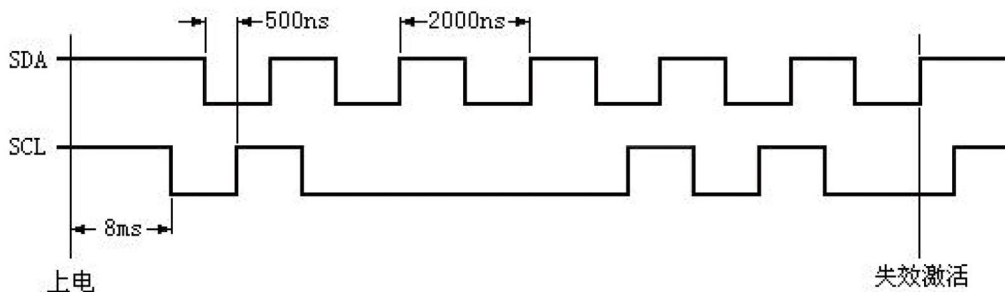
图9. POR失效时序图
