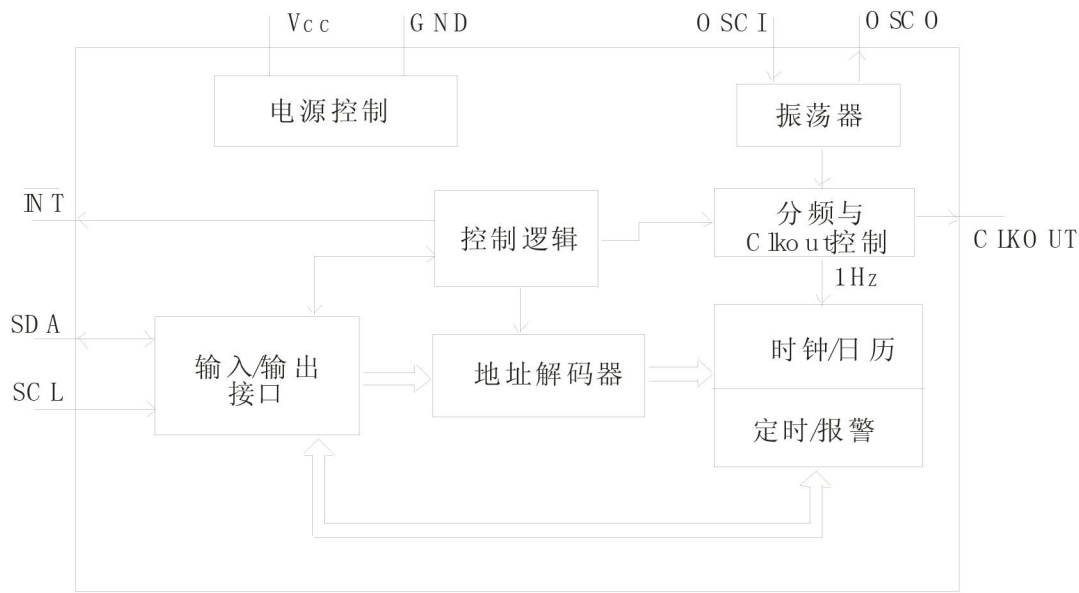
图 2. 方框图
