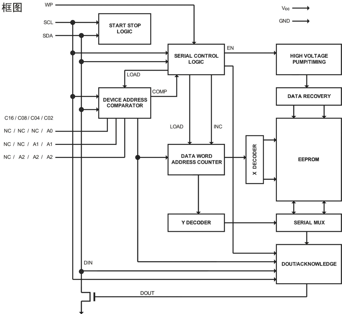
图1 框图
