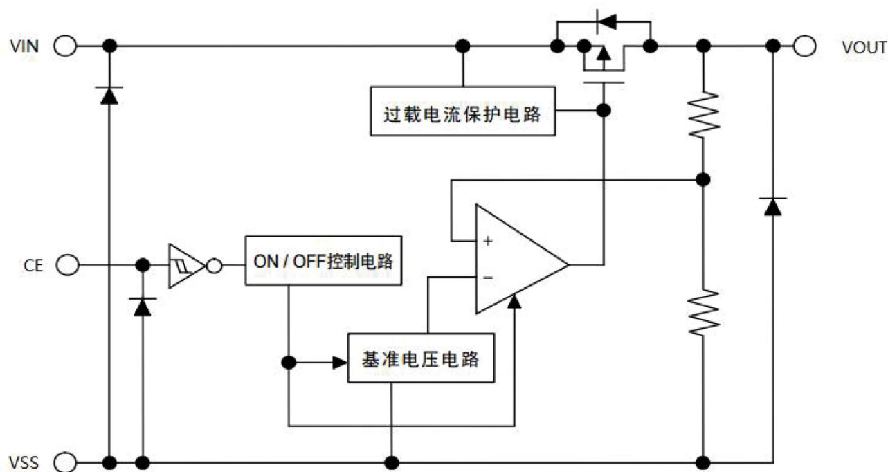
电路方框图
