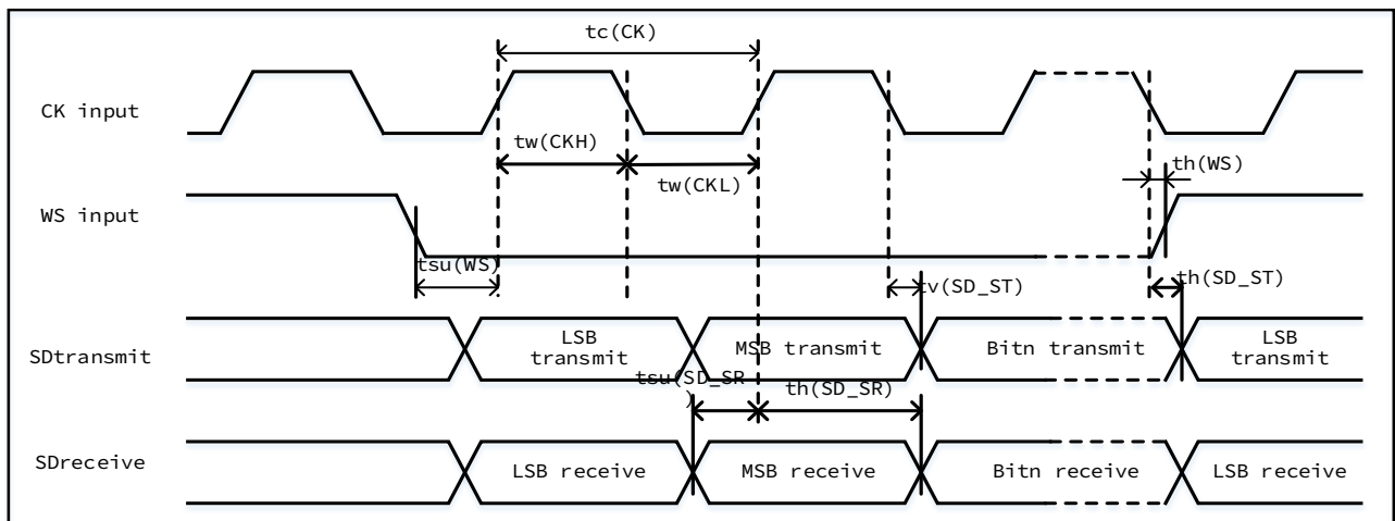
图 3-15 I2S 从模式时序 (Philips 协议)
