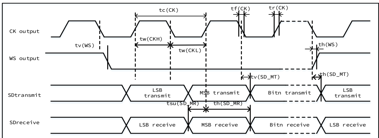
图 3-16 I2S 主模式时序 (Philips 协议)
