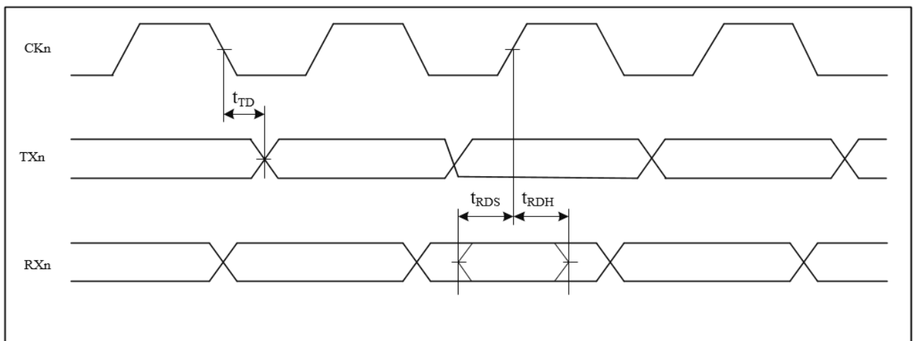
图 3-24 USART (CSI) 输入输出时序
