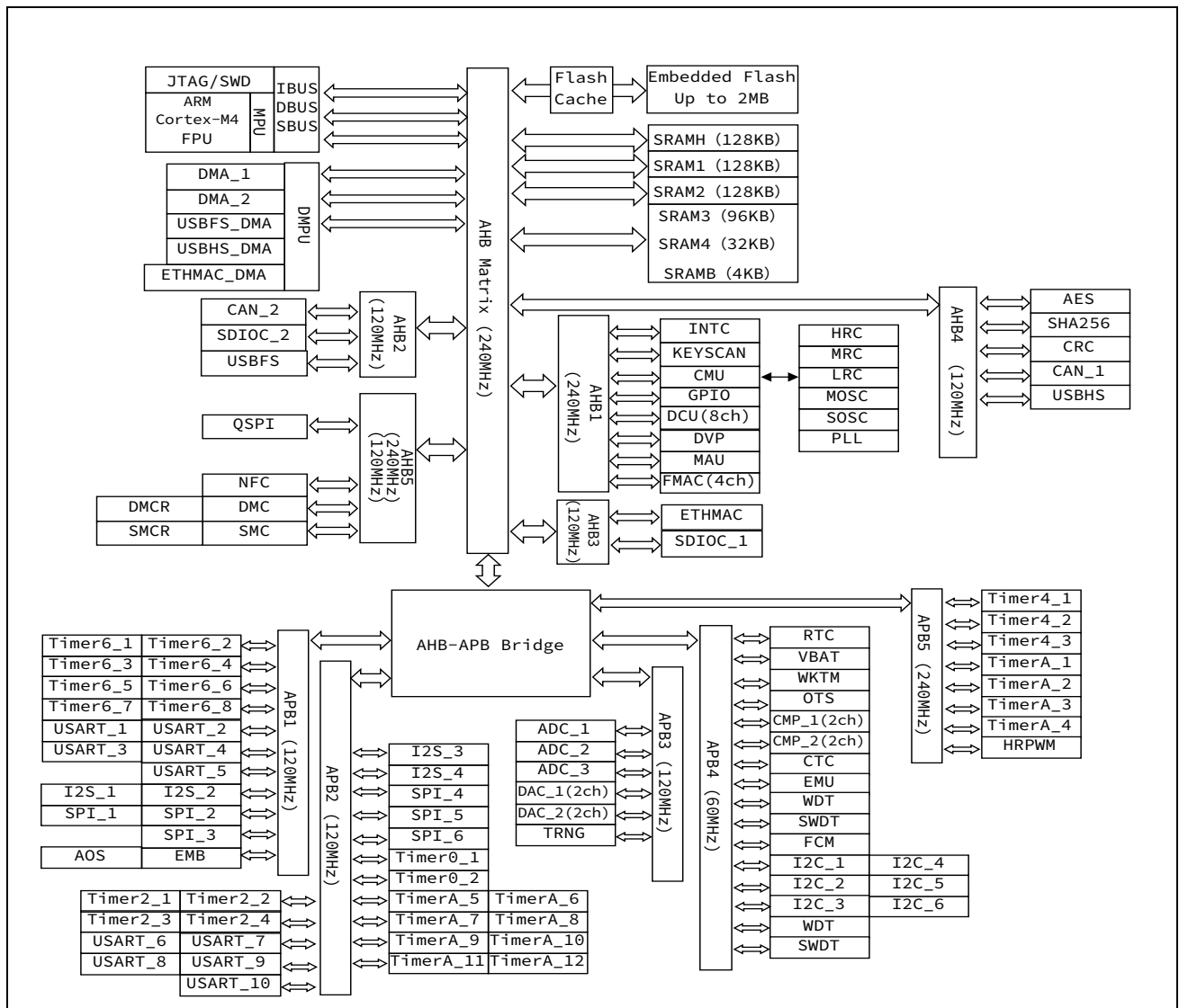
图 1-1 功能框图
