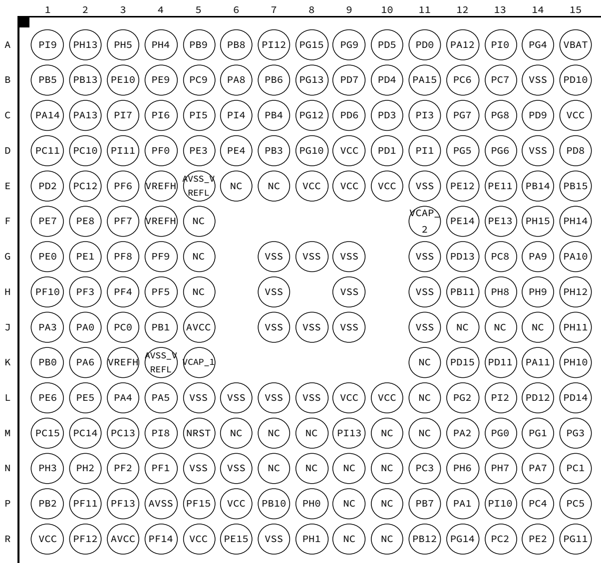
图 2-1 引脚配置图
