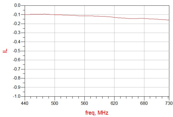
Figure 10. MHC0600L03 IL
