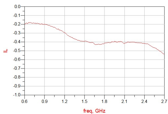
Figure 10. MHC0627L03 IL
