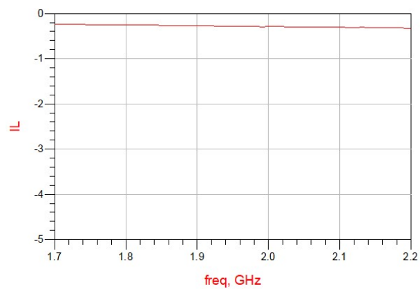
Figure 10. MHC2100L03 IL
