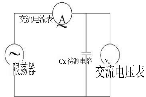
图3. 交流阻抗测试电路图
