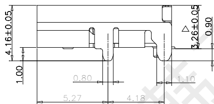
截面B-B
