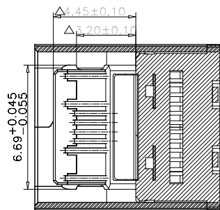
截面B-B
