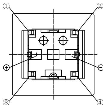
开关底部图
