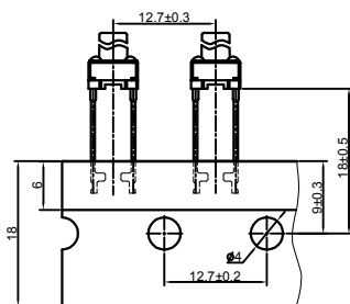
图1 编带图
