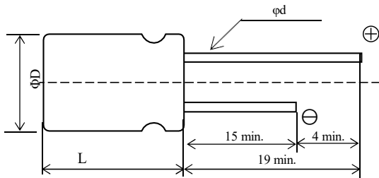
◆尺寸图 [mm]
