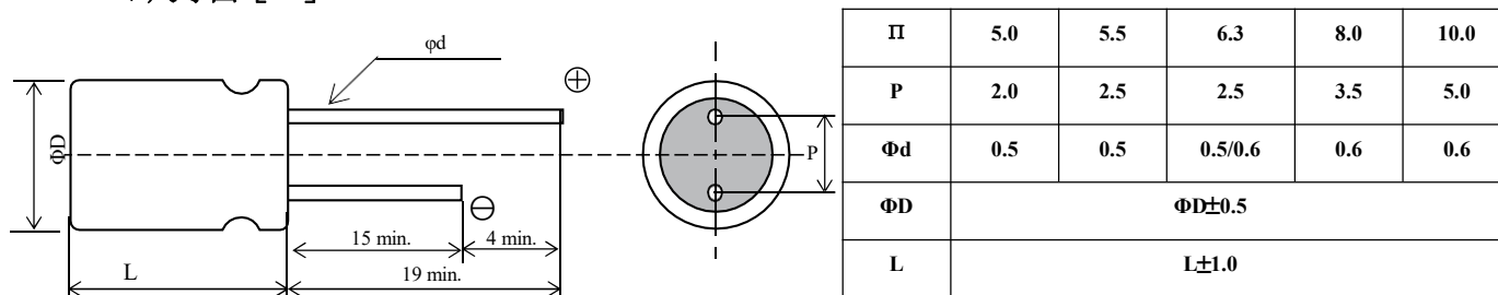
◆尺寸图 [mm]
