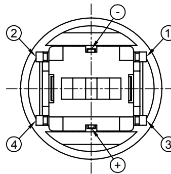
开关底部图
