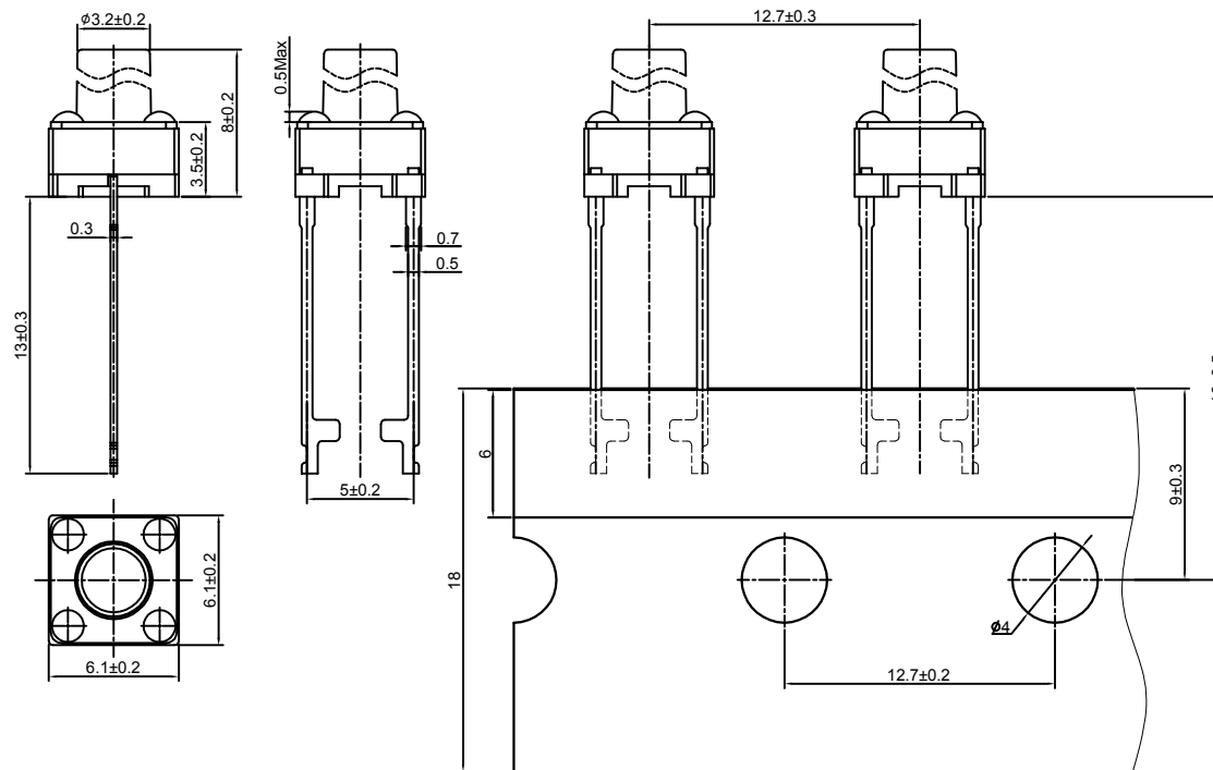
P.C.B. LAYOUT
