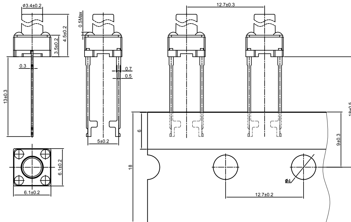
P.C.B. LAYOUT
