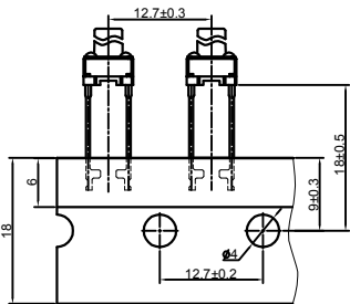
图1 编带图
