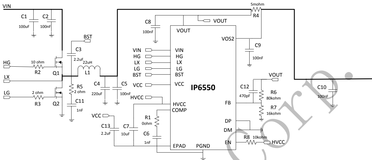
图9 IP6550_HV 外部反馈单口输出应用原理图
