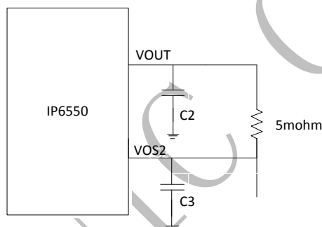
图 6 IP6550_HV 的输出限流电路图
