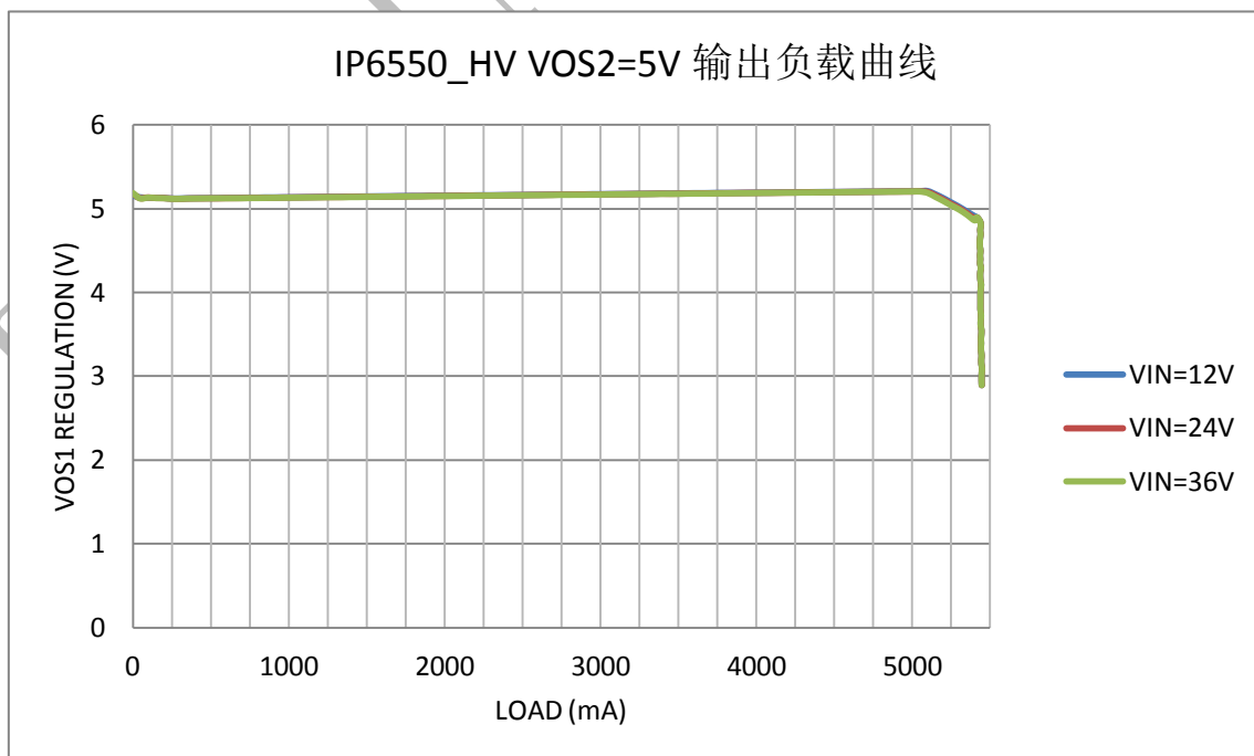
图 5 IP6550_HV VOS2-IOUT 曲线
