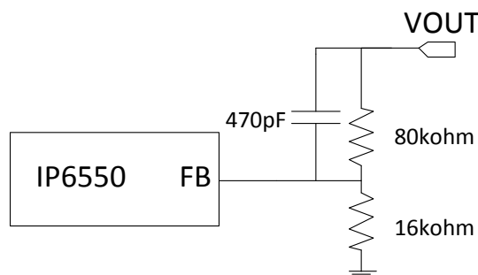
图 8 IP6550_HV 的 FB 反馈电路图
