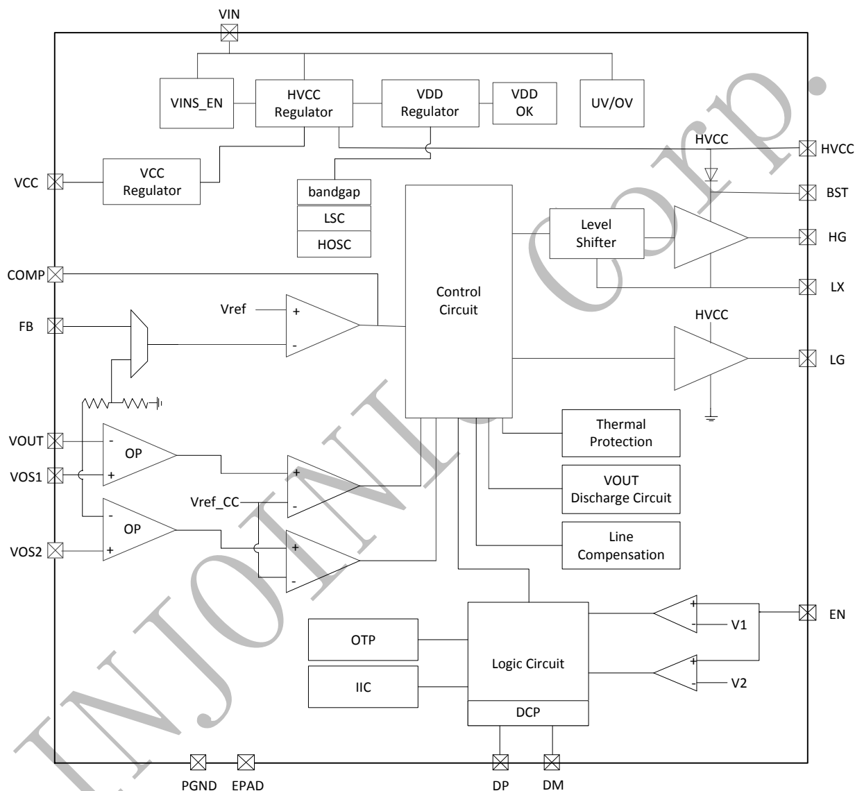
图 3 IP6550_HV 内部框图
