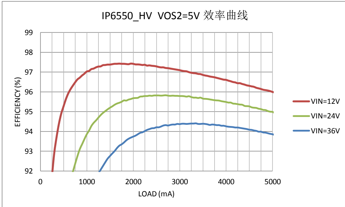
图 4 IP6550_HV VOS2 输出效率曲线
