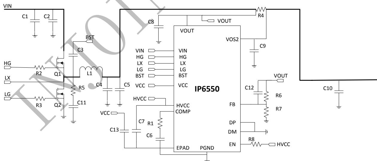
图 1 IP6550_HV 输出简化应用原理图
