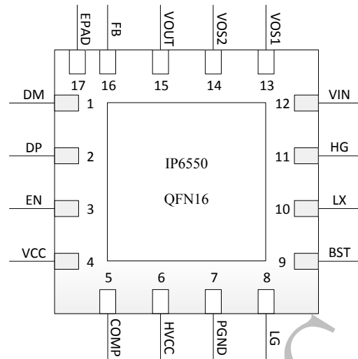
图 2 IP6550_HV 引脚图
