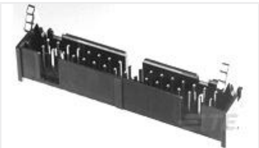
TE Part # 1761681-3 IDC LOW PRO HDR 10P VERT HT BLACK
