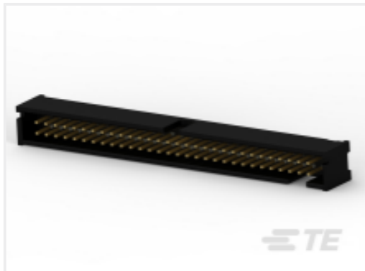
TE Part # 5103308-1 A/L LOW PRO HDR 10P VERT BLACK
