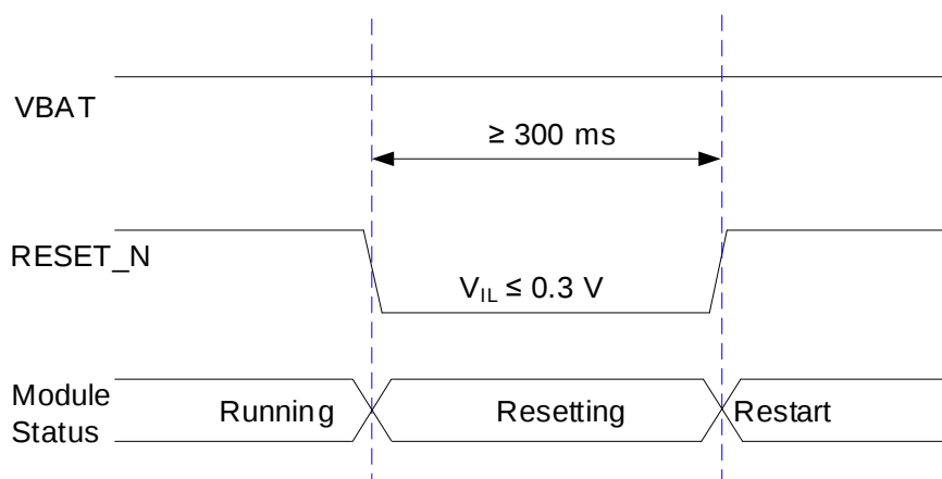
图 16: 复位时序图
