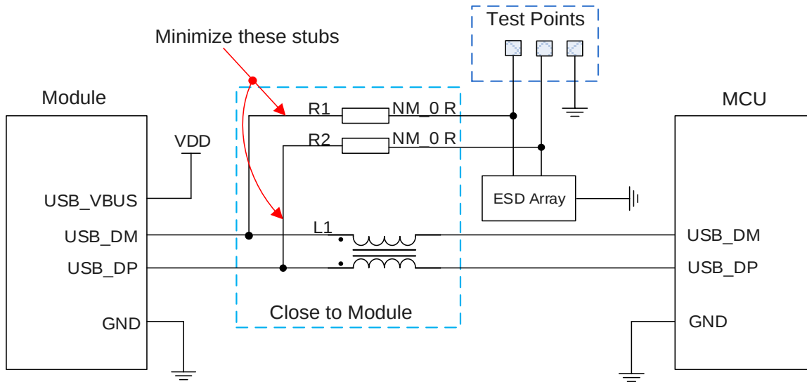
图 17: USB 接口参考电路图
