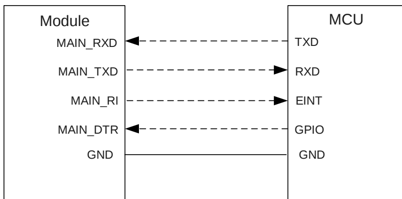
图 4：休眠模式下 UART 应用框图
