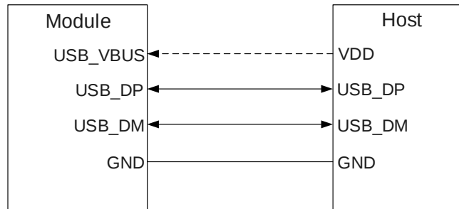
图 5：休眠模式下带 USB 远程唤醒功能的应用框图
