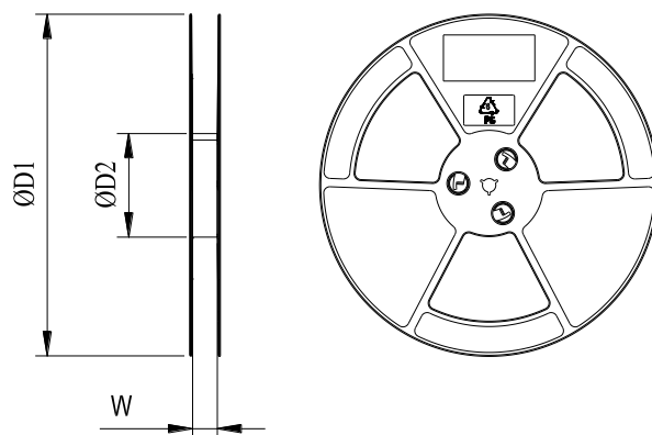
图 39: 胶盘尺寸图
