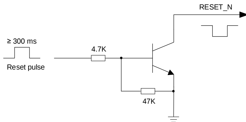
图 14: 开集驱动复位参考设计图
