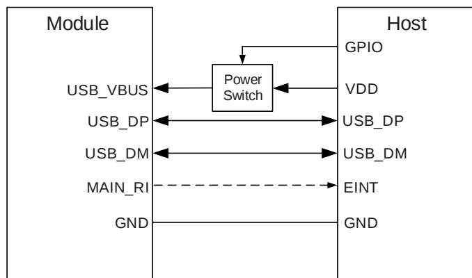
图 7：休眠模式下不支持 USB 挂起功能的应用框图
