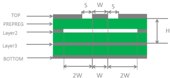
图 28: 四层 PCB 板共面波导结构（参考地为第三层）
