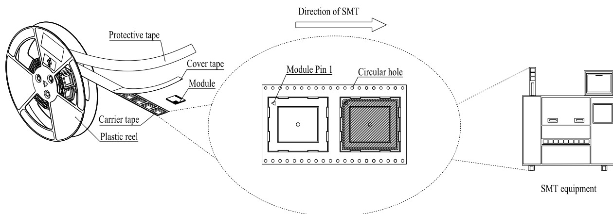
图 40: 贴片方向
