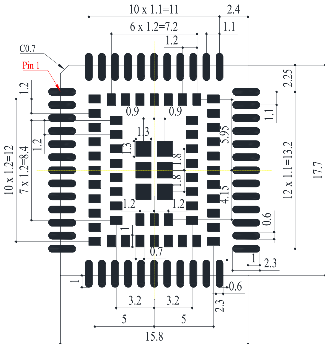
图 35: 推荐封装
