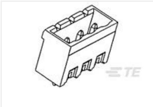
TE Part #796980-3 3 POS TERMI-BLOK VERT HDR 7.62
