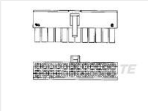
TE Part #1-794954-0 10P RCPT VAL-U-LOK V2
