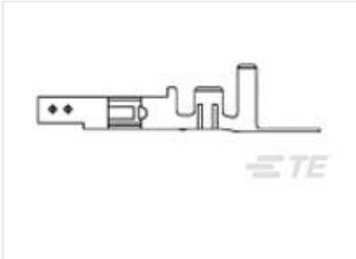
TE Part #794956-4 VAL-U-LOK SKT PHBZ AU 22-18AWG
