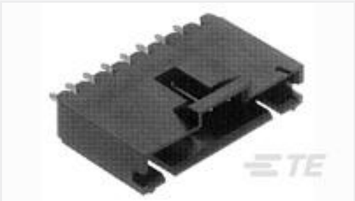
TE Part #NB17584001 RT-375-3/4-X-SP
