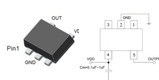
SOT-553
