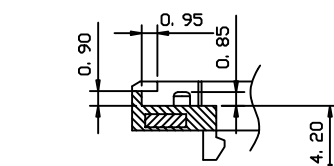
SECTION A-A SCALE 3:1
