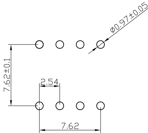
PCB开孔
