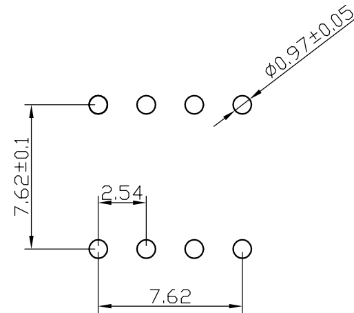
PCB开孔
