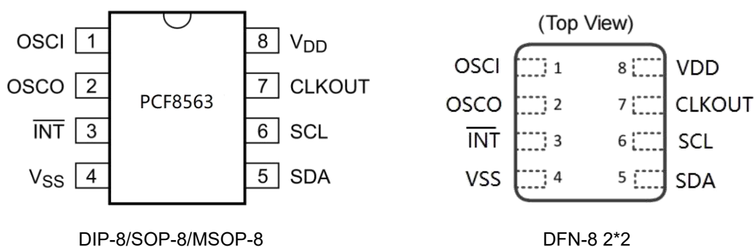
图 3 引脚图
